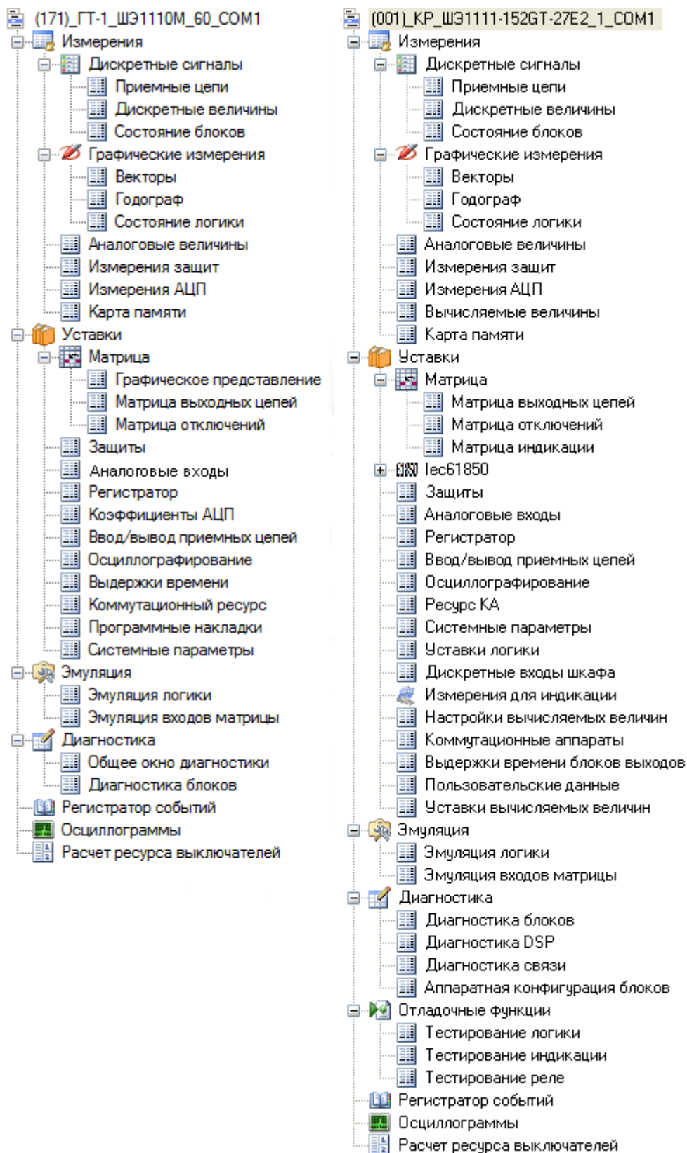
Рисунок 2.15 - Меню терминала (слева – 100-й серии, справа – 200-й серии)
